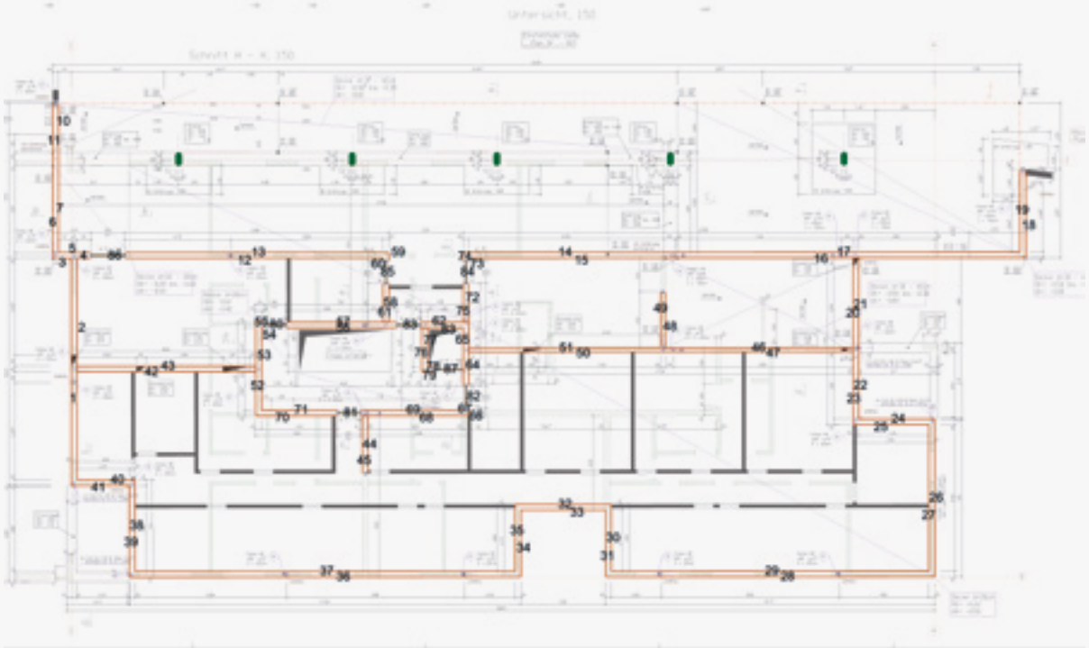
Grafikauszug einer Deckenschalung
